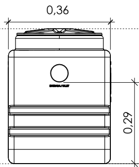
VISTA FRONTAL (entrada)
