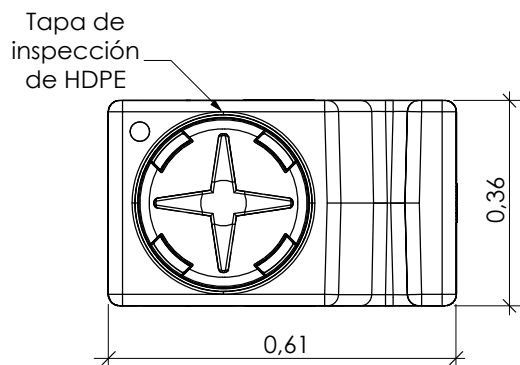
VISTA SUPERIOR
