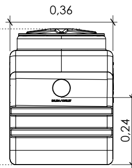
VISTA POSTERIOR (salida)
